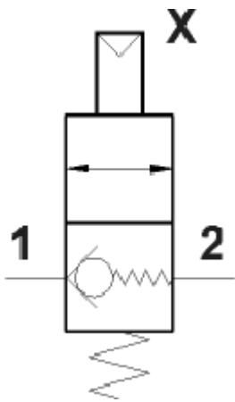
2/2 blokkeerventiel symbol
